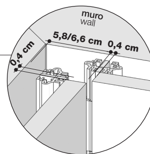
MATI montaggio ad angolo MATI corner setup
