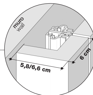
MATI profilo di chiusura MATI end filler
