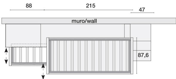
pianta plan
