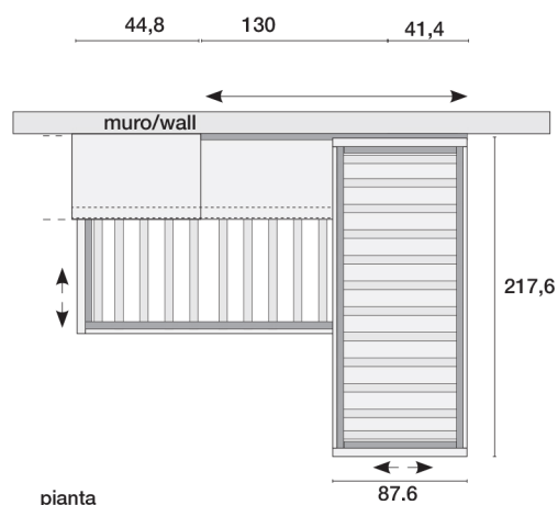
pianta plan
