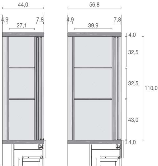
MODULO AD USO BAR BAR MODULE
