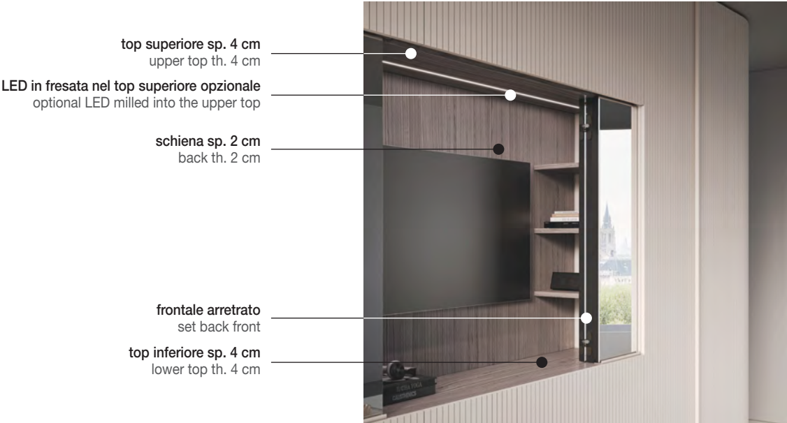
MODULO AD USO TV TV MODULE
